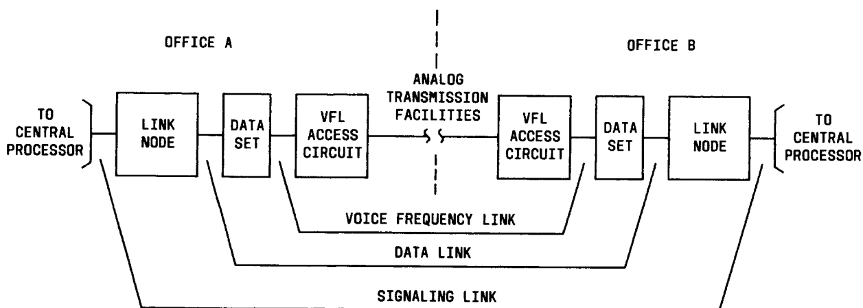
Fig. 2—Analog Signaling Link
