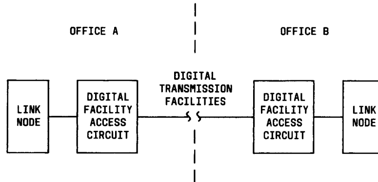
Fig. 4—56-Kbps Digital Signaling Link
