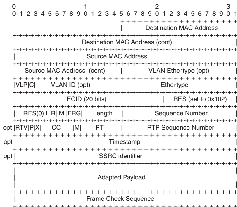
Figure 49 CESoETH Encapsulation
