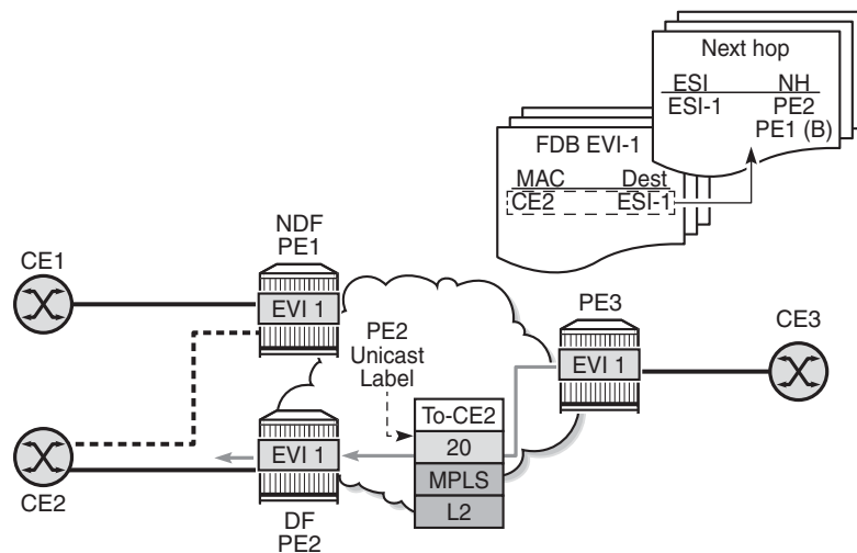
Figure 168 Backup PE
