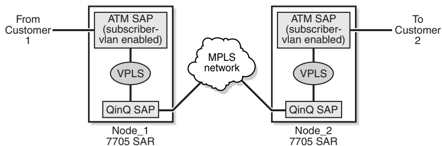
Figure 33 QinQ Using VPLS ATM SAPs
