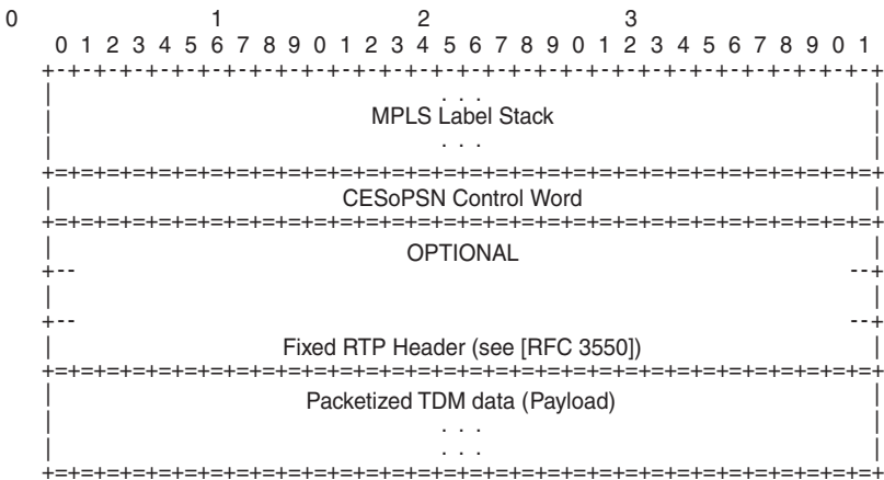
Figure 43 CESoPSN MPLS Encapsulation
