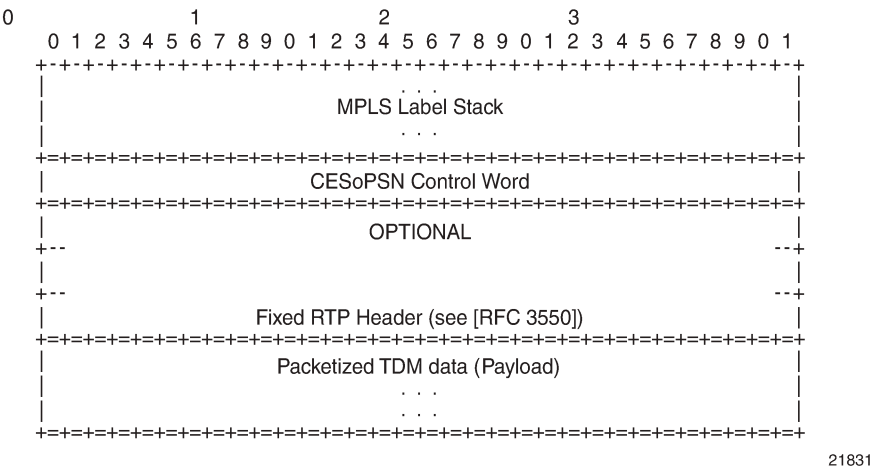
Figure 4: CESoPSN MPLS encapsulation
