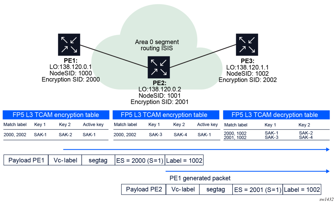
Figure 88: ANYsec encryption SID
